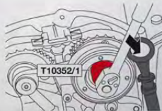
Engine Timing Tool Set for camshaft adjustment - VAG Juego de herramientas de ajuste de motores para ajuste de árboles de levas - VAG Jogo de ferramentas para ajuste de motores para desajuste de árvore de cames - VAG
